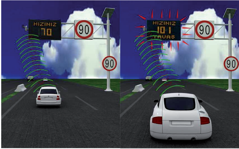
Şekil 5.1. LED’li radar panolarının çalışma prensibi
