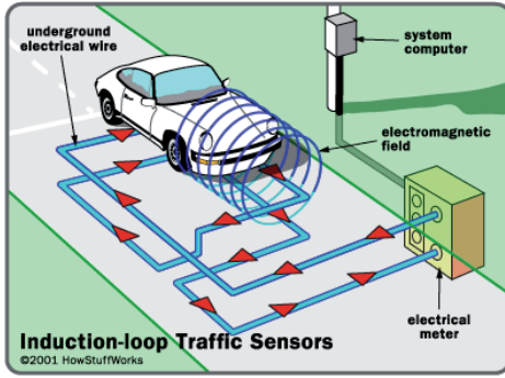
Şekil 3.2. Loop detektörlerin çalışma mantığı [4]
