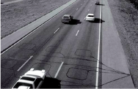
Resim 3.7. Loop detektörlerin asfalt altına monte edilmiş hali (A.B.D.) [5]
